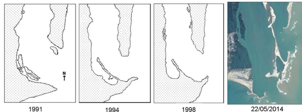
Figura 3: Alterações na geomorfologia da foz do rio Doce entre 1991 e 2014.
