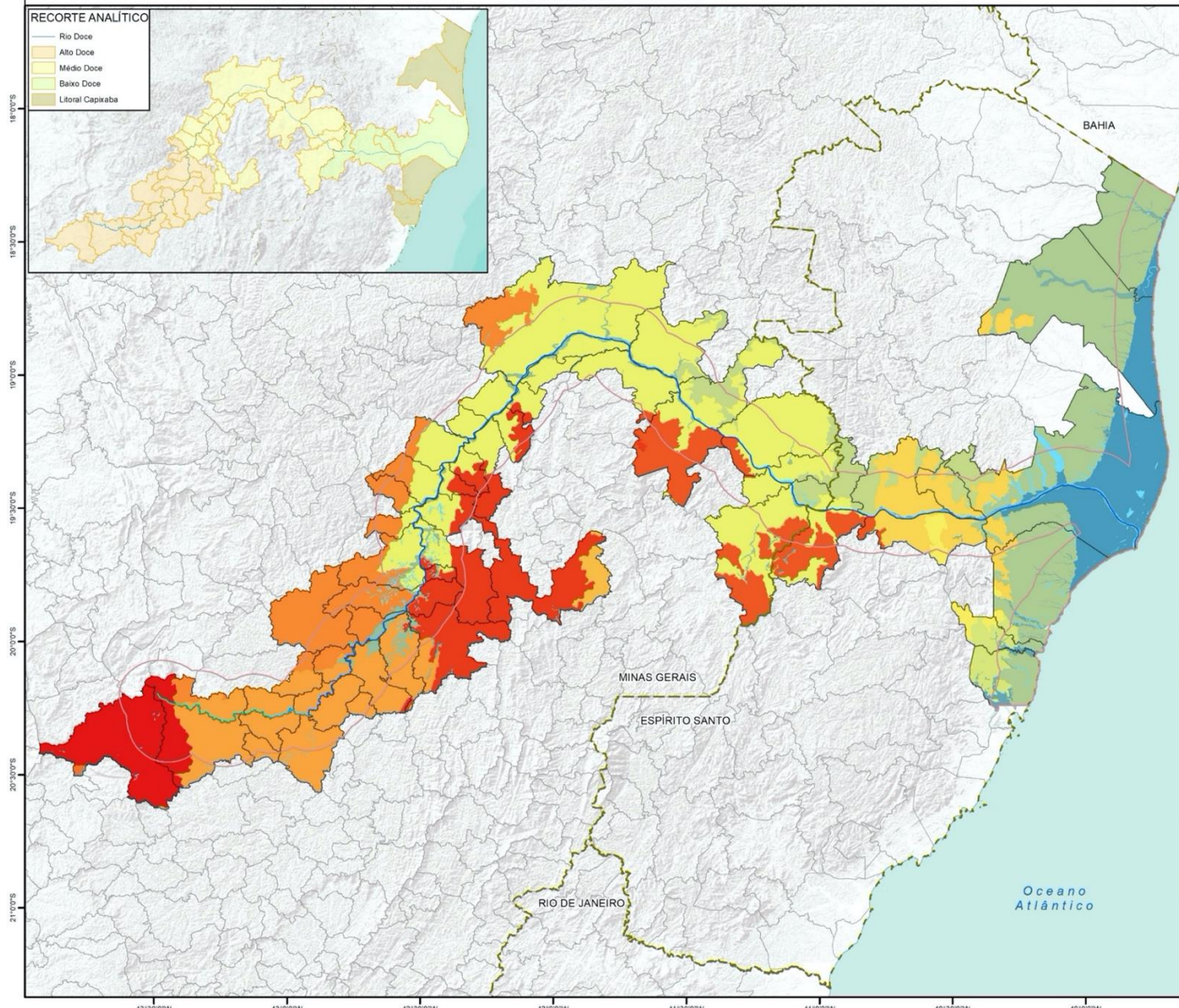
Mapa 6: Geomorfologia da área de estudo.
